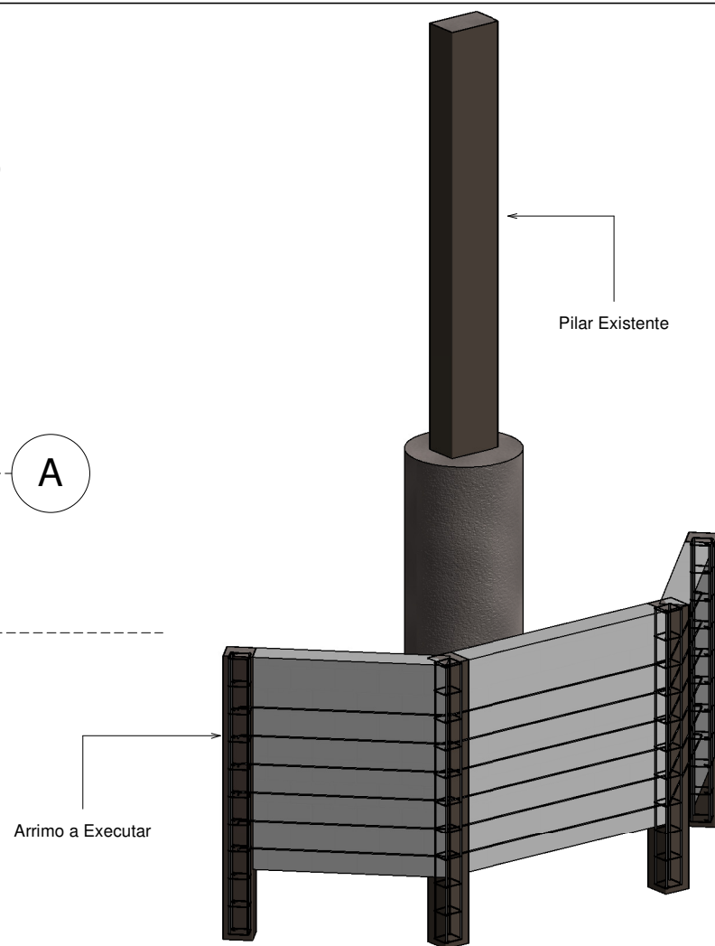
2 Vista Isométrica - 3D
