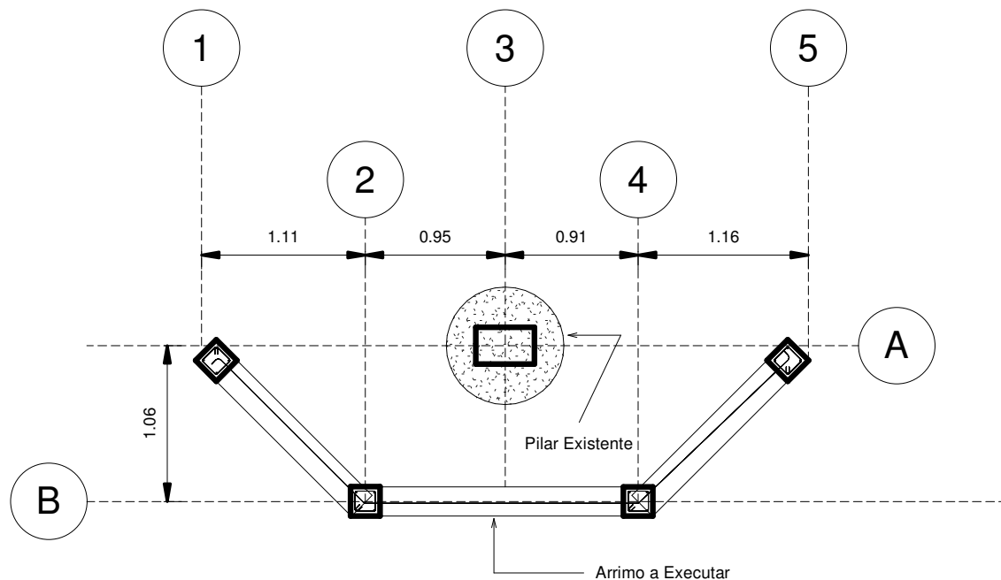
1 Planta Baixa 1 : 40
